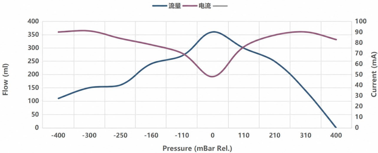
JSG13GE-KBD3-负载流量特性曲线(DC3.0V)
